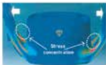
Konvenční rotor
